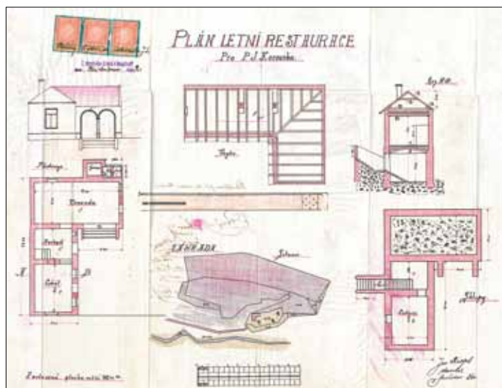
Plán přestavby restaurace Zátíší pro pana Kocourka z 30. dubna roku 1902
